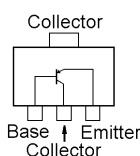
2SB1301 (ZQ) (Q1511) 2SD1368CB (CB) (Q1504)
